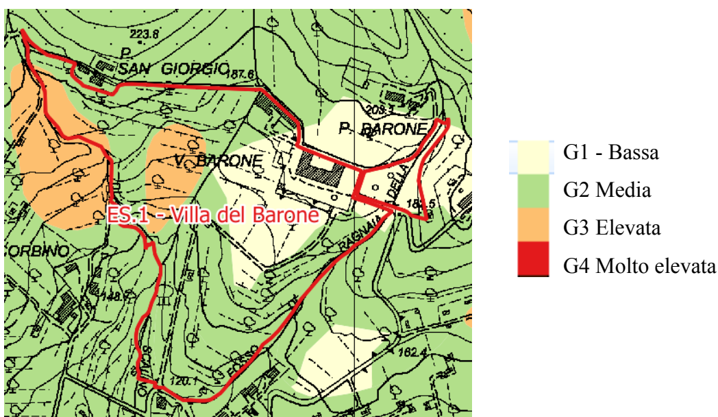
Fig. 1 – Dettaglio della Carta di Pericolosità Geomorfológica del PS
